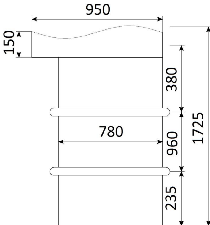
Рисунок 1 – Габариты фильтра
